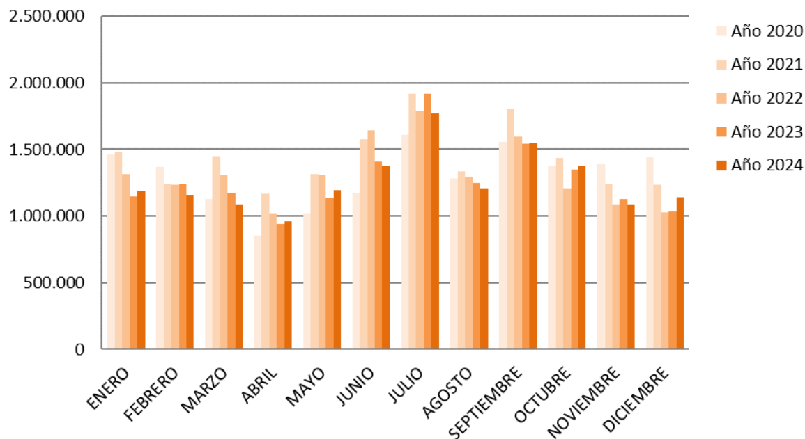
Consumo de Electricidad por Mes en la UMH
