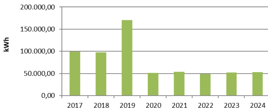
Generación de kWh por Biomasa en la UMH
